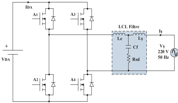
Şekil 1: LCL filtreli bir fazlı evirici devresi.
