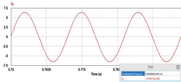
Şekil 9: L_s = 3,9 mH değerinde iken şebeke akımı.
